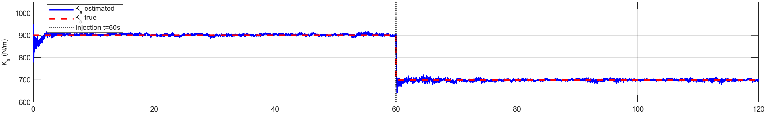
Spring Stiffness K_s — AEKF Parameter Estimation
